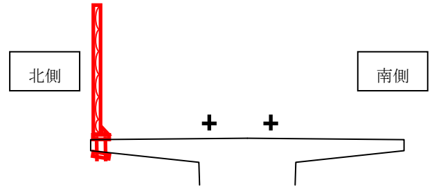
橋りょう区間標準断面図
